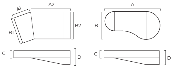
Lazy en pente composée (avec ou sans marche de sécurité)
