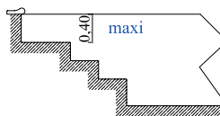
La coupe
