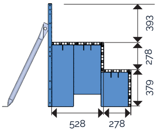
H.1,06m - 2 marches
