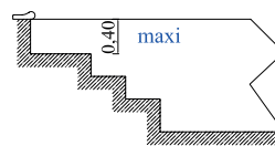
La coupe
