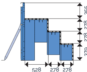
H.1,30m - 3 marches
