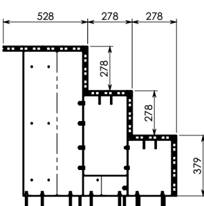
H.1,30m - 3 marches
