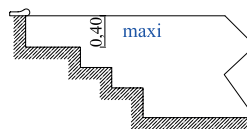
La coupe
